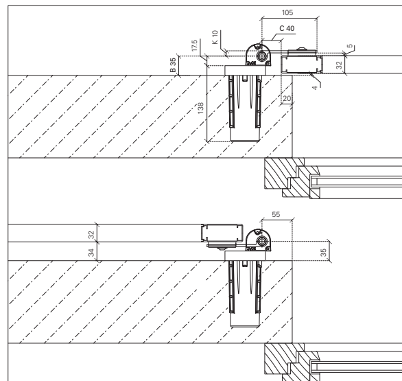
Montageart 4: aufliegend
