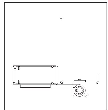
ohne Falzleiste
