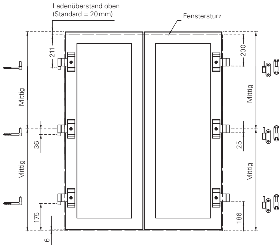
Montageart 4 (aufliegend)
