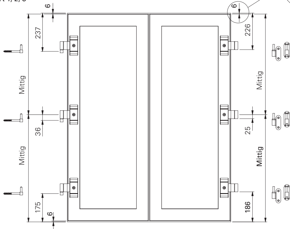
Montageart 1, 2, 3
