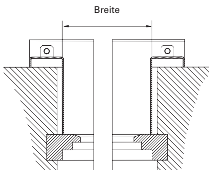
ohne Flügel
