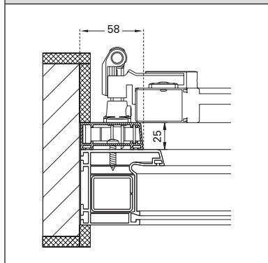
C (eingeputzt oder seitlich bündig)
