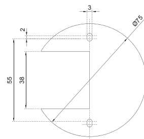
Motorabdeckung
