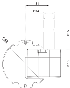
Klobenantrieb
