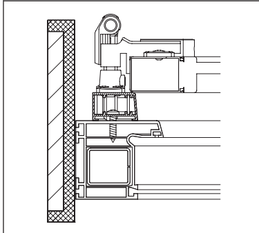
B (von außen verschraubt)
