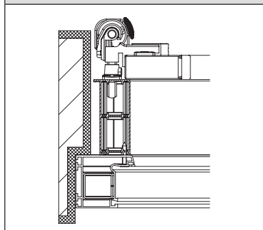
C (mit Rasthalter von innen verschraubt)
