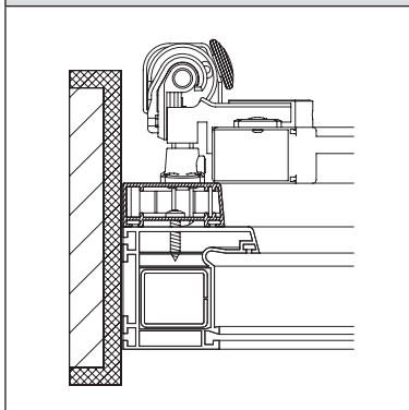
B (mit Rasthalter seitlich bündig)
