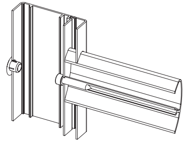
Querfries, verdeckt
