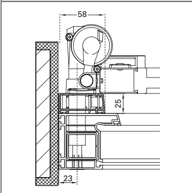
A (mit Innenöffner seitlich bündig)
