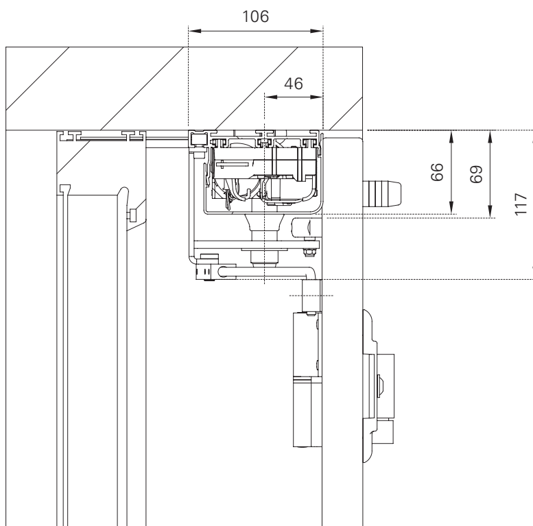
Ausführung mit Doppelladen
