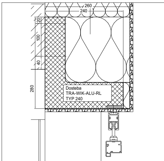
Klobentrageelement TRA-WIK-ALU-RL
