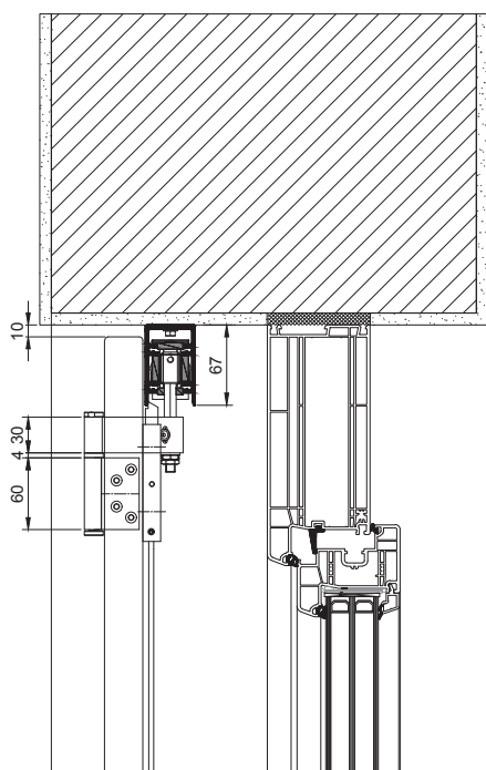
Typ A Sturz | Type A
