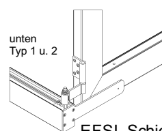
EFSL Schienenendanschlag
