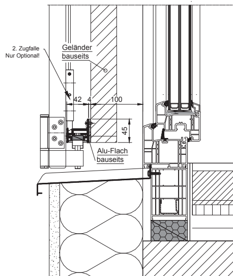
Typ 1 Geländer | Type 1
