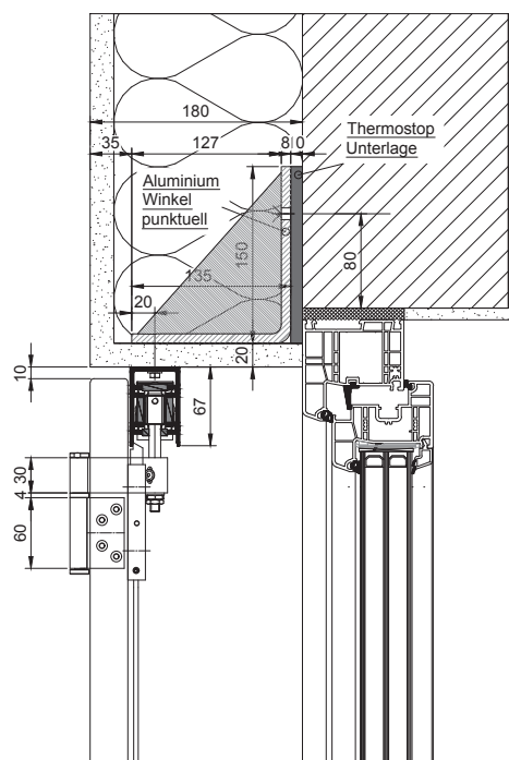
Typ A Konsole | Type A
